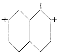
Bender. Ber. 22. 996.
